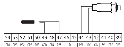
Connessione sonda di temperatura + sonda di pressione
