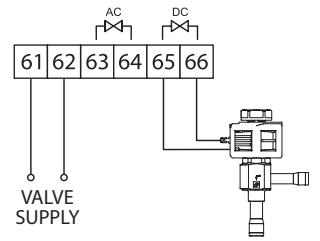
Connessione valvola DC
