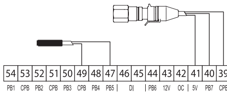
Connessione sonda di temperatura + sonda raziometrica
