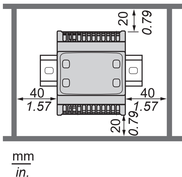
Рис. 7. Расстояния до стенок щитка
