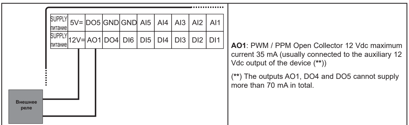
Рис. 21. Пример подключения внешнего реле на выход AO1 (Открытый коллектор) EWCM 436D PRO STD
