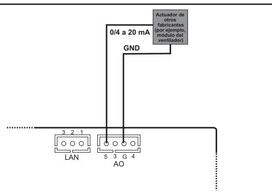
Fig. 23. Ejemplo conexión EWCM 436D PRO A-STD (AO5) con 1 módulo ventiladores 0...20 mA / 4...20 mA
