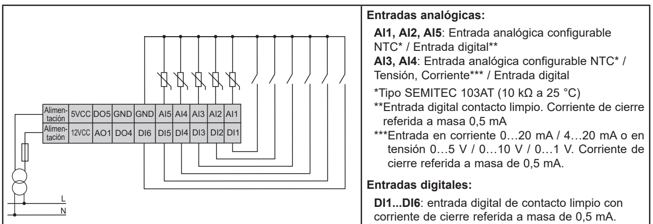
Fig. 20. Ejemplo conexión entradas analógicas / digitales
