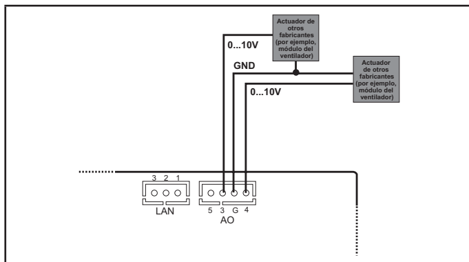
Fig. 22. Ejemplo conexión EWCM 400D PRO A-STD (AO3-AO4) con 1 módulo ventiladores 0...10 V
