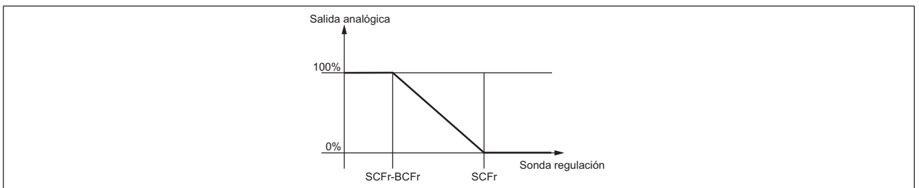
Fig. 44. Regulador genérico salida analógica - Modo Calor
