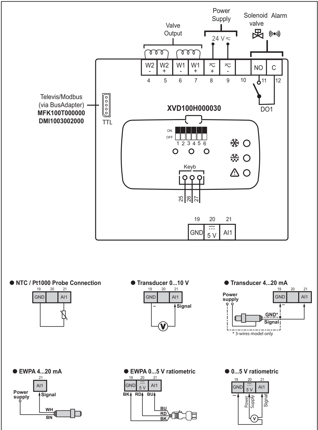
Fig. 11. Schema cablaggio XVD 100H ACTUATOR
