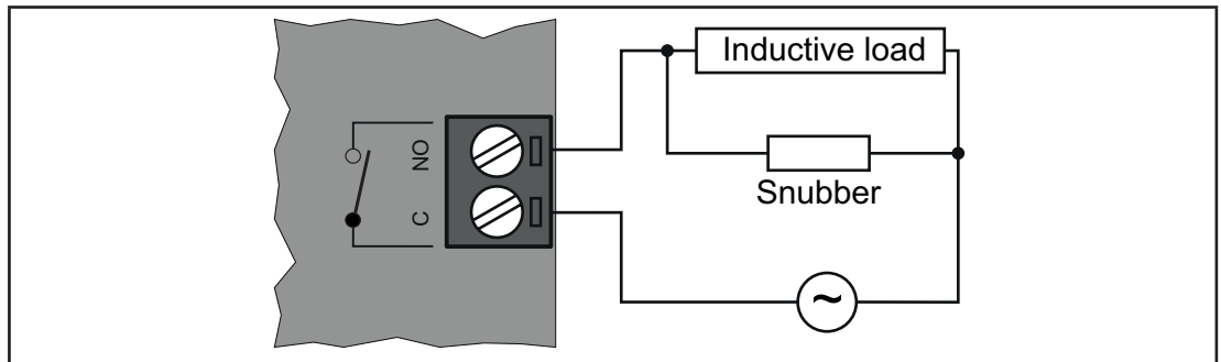
Fig. 6. Circuito di protezione A
